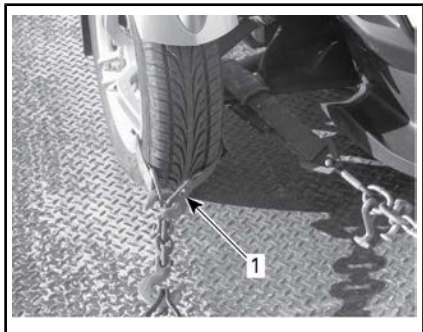
AGGANCIAMENTO RUOTE ANTERIORI — CONFIGURAZIONE TIPICA
