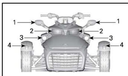
POSIZIONE DELLE LUCI — DAVANTI DEL VEICOLO — MODELLI EUROPEI, BRASILIANI, AUSTRALIANI E GIAPPONESI
