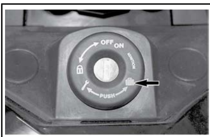
POSIZIONE DELLA CHIAVE PER L'APERTURA DELLO SCOMPARTO ANTERIORE
