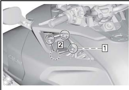
Fase 1: Rimuovere le quattro viti Fase 2: Rimuovere il coperchio del filtro dell'aria
