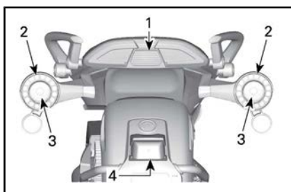
POSIZIONE DELLE LUCI — RETRO DEL VEICOLO — MODELLI GIAPPONESI
