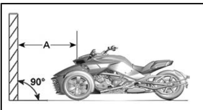
CONFIGURAZIONE TIPICA - RIFLESSO DEI FARI SULLA SUPERFICIE DI PROVA — ABBAGLIANTE (FARO SINGOLO)
