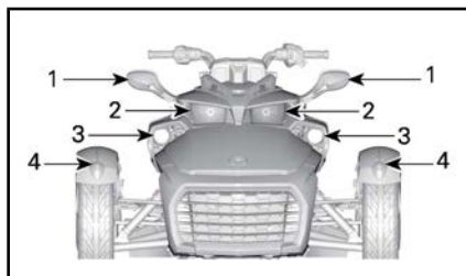
CONFIGURAZIONE TIPICA - POSIZIONE DELLE LUCI - PARTE ANTERIORE DEL VEICOLO - MODELLI NORDAMERICANI
