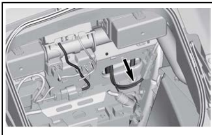
DC12 - CIRCUITO ACCESSORIO DEL CLIENTE ANTERIORE - DIETRO LO SCOMPARTO ANTERIORE
