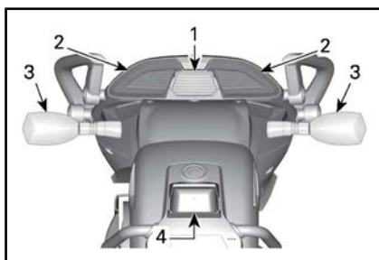
POSIZIONE DELLE LUCI — RETRO DEL VEICOLO — TUTTI I MODELLI AD ECCEZIONE DEI MODELLI NORDAMERICANI E GIAPPONESI
