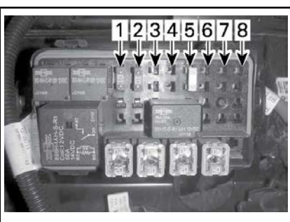
FUSIBILI - SCATOLA FUSIBILI DESTRA
