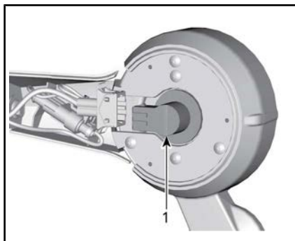
1. Gire el portalámparas para liberarlo.
