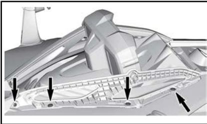
TORNILLOS DE SUJECIÓN QUE DEBEN QUITARSE
