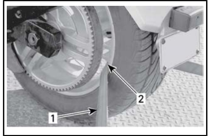
TÍPICO - SUJECIÓN DE LA RUEDA TRASERA
