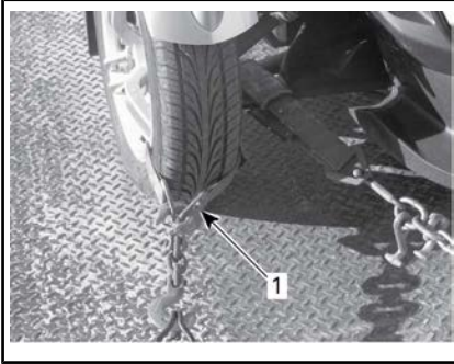
TÍPICO - SUJECIÓN DE LAS RUEDAS DELANTERAS
