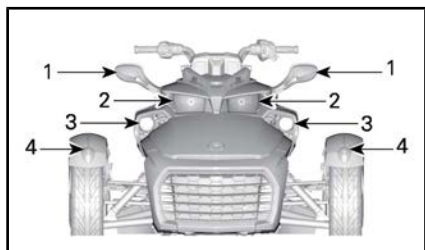
UBICACIÓN TÍPICA DE LAS LUCES: PARTE DELANTERA DEL VEHÍCULO (MODELOS NORTEAMERICANOS)
