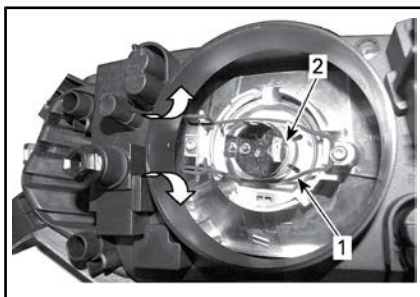
1. Muelle de retención de la lámpara
