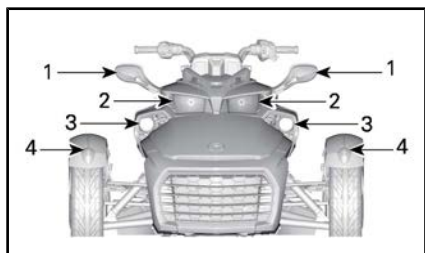
UBICACIÓN DE LAS LUCES - PARTE DELANTERA DEL VEHÍCULO (MODELOS EUROPEOS, AUSTRALIANOS Y JAPONESES)
