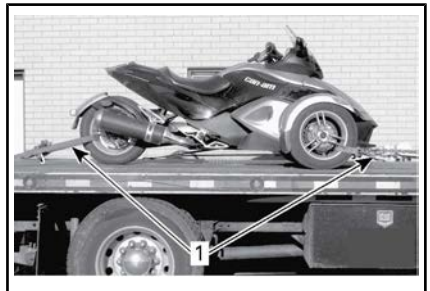
TÍPICO - REMOLCADO CON EL VEHÍCULO ORIENTADO HACIA ADELANTE
