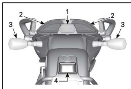
UBICACIÓN DE LAS LUCES — PARTE TRASERA DEL VEHÍCULO (TODOS LOS MODELOS EXCEPTO LOS NORTEAMERICANOS Y JAPONESES)
