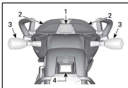
TYPISCH - PLAATSING VAN DE LICHTEN — ACHTERAAN HET VOERTUIG — ALLE MODELLEN BEHALVE NOORD-AMERIKAANSE EN JAPANESE LIMITED- EN T-MODELLEN
