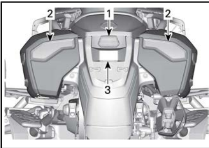
TYPISCH - LOCATIE LICHTEN - ACHTERKANT VAN HET VOERTUIG - LIMITED-EN T-MODELLEN - ALLE LANDEN
