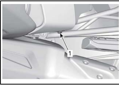
1. Plastic klinknagel bovenop de zadeltas
