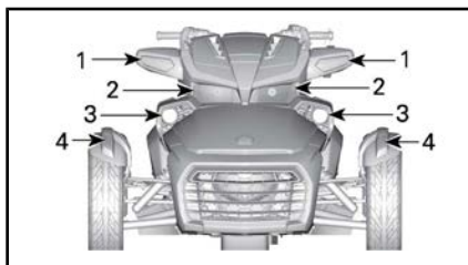
TYPISCH - PLAATSING VAN DE LICHTEN — VOORAAN HET VOERTUIG — EUROPESE, AUSTRALISCHE EN JAPANESE T-EN LIMITED-MODELLEN
