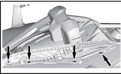
TYPISCH - TE VERWIJDEREN BORG-SCHROEVEN
