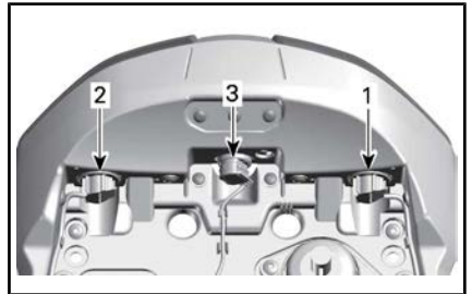
1. Verwijder de richtingaanwijzerconnector
