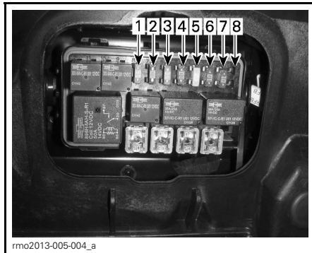
FUSIBLES - BOÎTE À FUSIBLES DROITE
