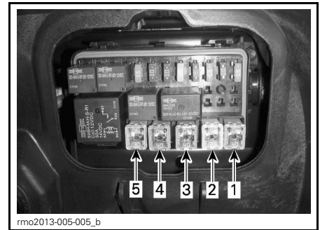
FUSIBLES JCASE - BOÎTE À FUSIBLES GAUCHE
