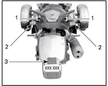
TÍPICO: UBICACIÓN DE LAS LUCES — PARTE TRASERA DEL VEHÍCULO
