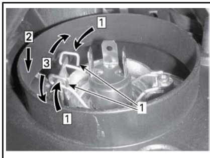
1. Pasador de retención
