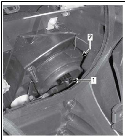
1. Conector eléctrico 2. Manguito de goma
