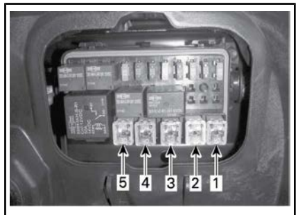
J-KASTEN-SICHERUNGEN - LINKER SICHERUNGSKASTEN
