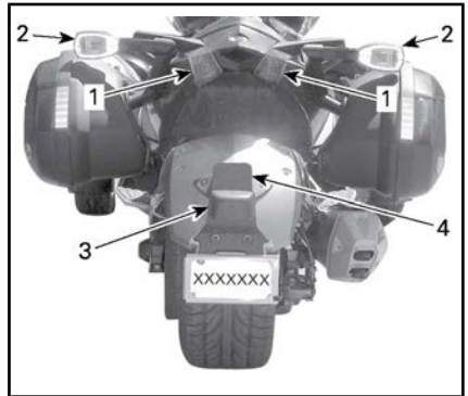
TYPISCH - LEUCHTENANORDNUNG — FAHRZEUGRÜCKSEITE
