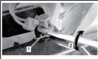
1. Flachkopf-Schraubendreher unter dem Niet 2. Schraubendreher eine Viertelumdrehung drehen 3. Lösen Sie die Stecker vom rechten Blinkergehäuse. 4. Entfernen Sie die Torx-Schraube hinter dem Glas wie unten dargestellt.
