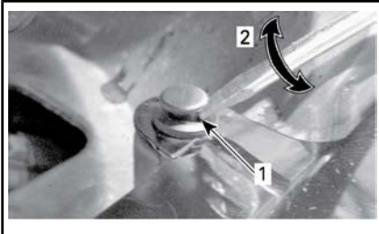
1. Flachkopf-Schraubendreher unter dem Nietkopf 2. Schraubendreher eine Viertelumdrehung drehen
