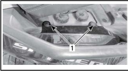
1. 2 Kunststoffniete unter dem Sitz
