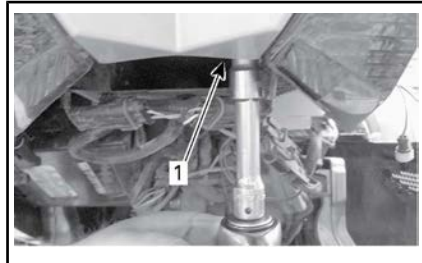
1. Entfernung der Torx-Schraube neben dem Glas
