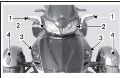
TYPISCH - LEUCHTENANORDNUNG — FAHRZEUGVORDERSEITE
