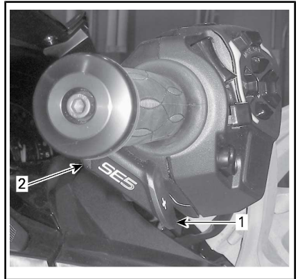
1. Innesto marcia alta 2. Innesto marcia bassa
