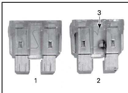
FUSIBILI A CAPSULA - SCATOLA FUSIBILI DESTRA
