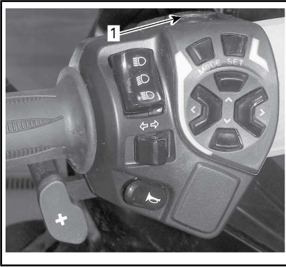
1. Pulsante della retromarcia
