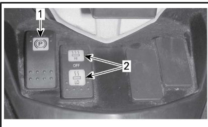
1. Interruttore freno stazionamento 2. Interruttore manopole riscaldate conducente (pacchetto opzionale)
