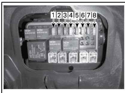
FUSIBILI - SCATOLA FUSIBILI SINISTRA
