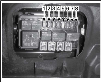
FUSIBILI - SCATOLA FUSIBILI DESTRA
