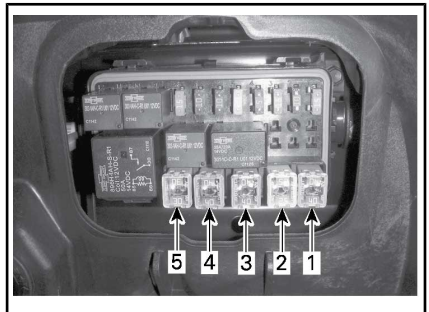
FUSIBLES JCASE - CAJA DE FUSIBLES IZQUIERDA
