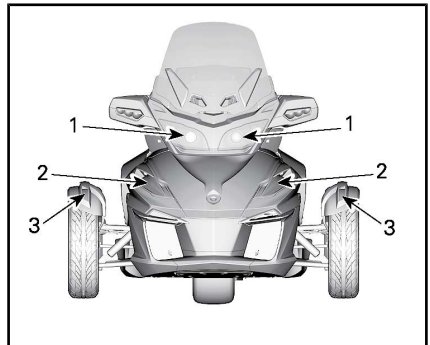
TYPISCH - LOCATIE LICHTEN — VOORKANT VAN HET VOERTUIG
