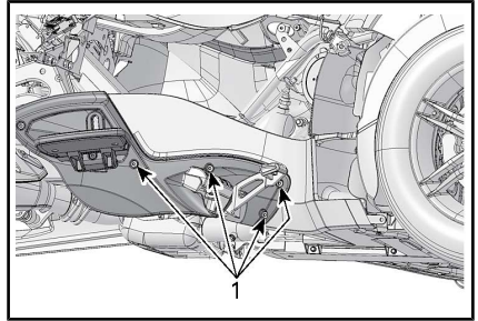
1. Borgschroeven
