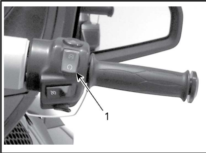
1. Motorstopschakelaar
