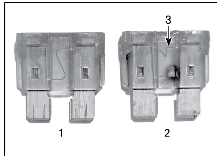
ZEKERING
