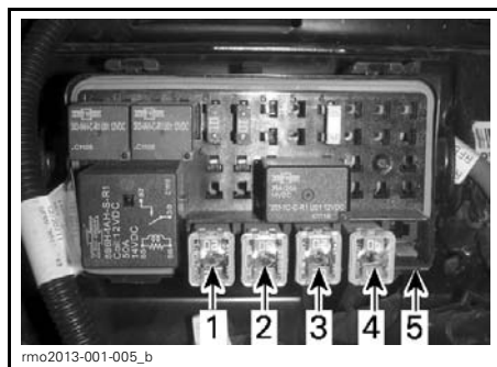
FUSIBLES JCASE - BOÎTE À FUSIBLES DROITE
