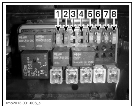
FUSIBLES - BOÎTE À FUSIBLE GAUCHE
