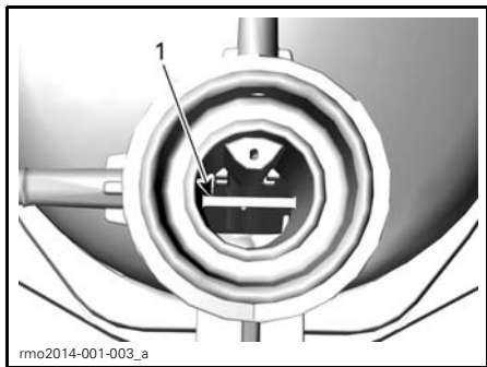
1. Ligne de référence du niveau de liquide de refroidissement (marque «HOT»)
