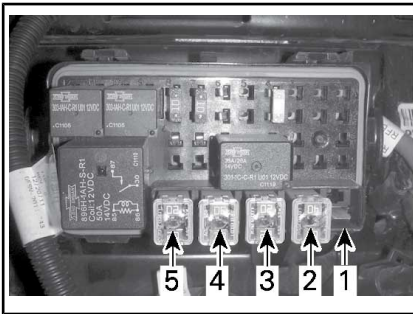
FUSIBLES HEMBRA: CAJA DE FUSIBLES DERECHA
