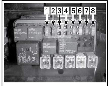
FUSIBLES: CAJA DE FUSIBLES IZQUIERDA
