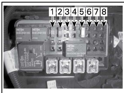
FUSIBLES: CAJA DE FUSIBLES DERECHA
