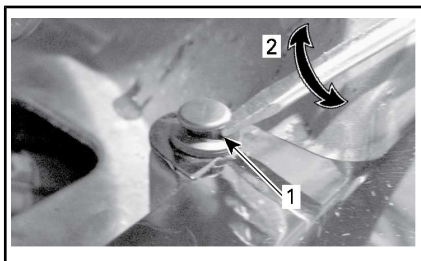
1. Remaches de plástico (2) bajo el asiento
