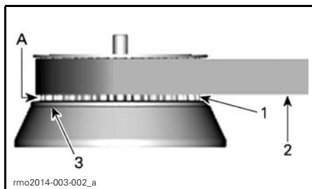
1. Dents du pignon avant 2. Courroie 3. Épaulement interne du pignon A. JEU "X"
