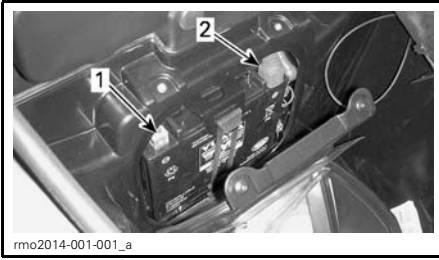
1. Borne NÉGATIVE (-) 2. Borne POSITIVE (+)
