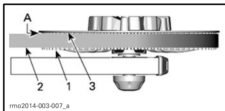
1. Dents du pignon arrière 2. Courroie 3. Épaulement interne du pignon A. JEU "Y"
