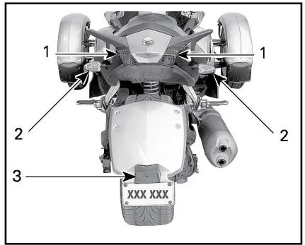
TÍPICO - UBICACIÓN DE LAS LUCES; PARTE TRASERA DEL VEHÍCULO
