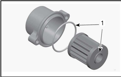
1. Aplique aceite aquí
