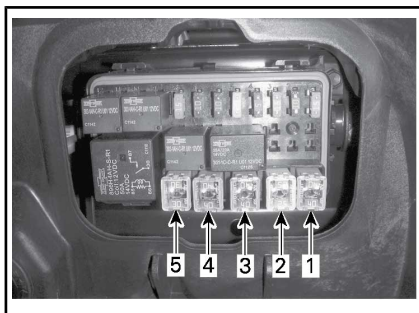
FUSIBLES JCASE - CAJA DE FUSIBLES IZQUIERDA
