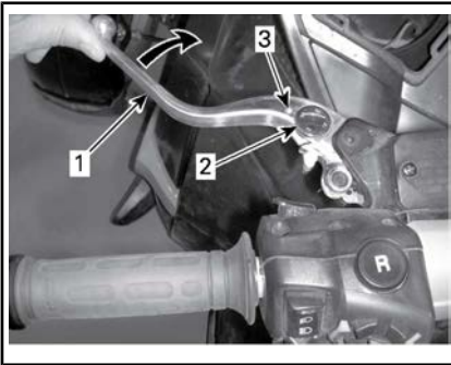
クラッチレバーの調整
