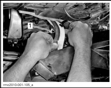
VISTA DE LA PARTE DERECHA
