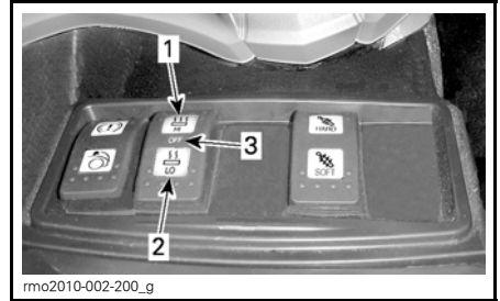
1. Alta intensidad (HI) 2. Baja intensidad (LO) 3. APAGADO (posición intermedia)
