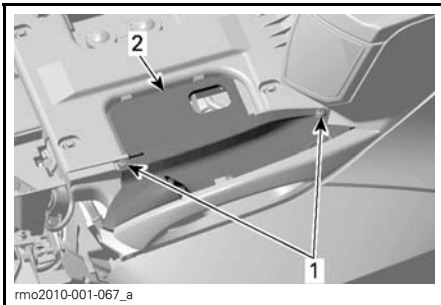
VISTA DEL PANEL LATERAL IZQUIERDO
