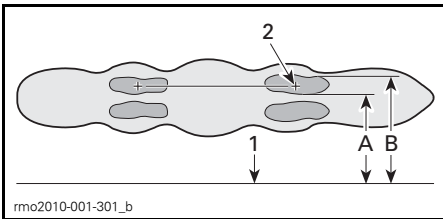
REFLEJO TÍPICO DE FAROS EN LA SUPERFICIE DE PRUEBAS
