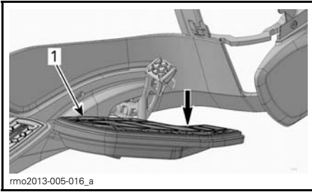
rmo2013-005-016_a PLACA DEL SUELO CON ALTURA REDUCIDA 1. Placa de suelo
