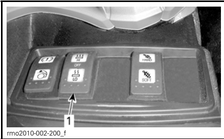
1. Interruptor de empuñaduras con calefacción
