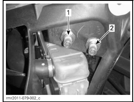
VISTA DE LA PARTE DERECHA
