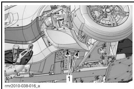
1. Trykklips
