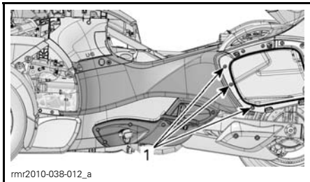
1. Bakre festeskruer
