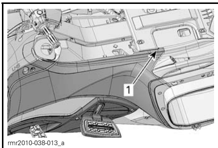
1. Øvre festeskruer
