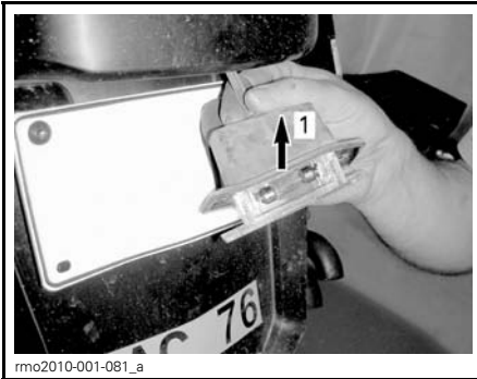
1. Trekk utover
