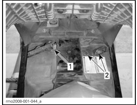
1. Borne NÉGATIVE (-) 2. Borne POSITIVE (+)
