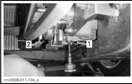
1. Bouchon de vidange d'huile à moteur 2. Couverture du filtre à huile
