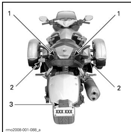
EMPLACEMENT DES FEUX — ARRIÈRE DU VÉHICULE
