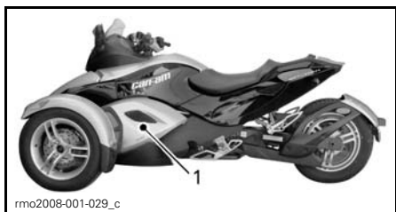
1. Étiquette 4 sur le réservoir d'huile derrière le panneau latéral central gauche
