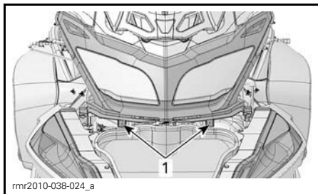
1. Vis de fixation inférieure
