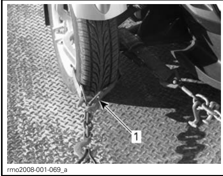
TYPIQUE - ARRIMAGE DES ROUES AVANT - METHODE 1
