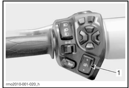
1. Bouton de réglage du pare-brise
