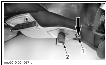
1. Pédale de frein 2. Repose-pied
