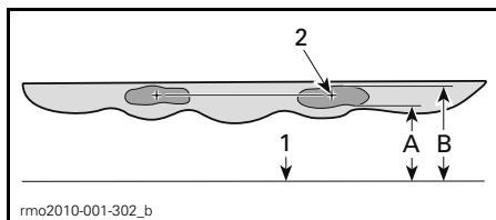
RÉFLEXION TYPIQUE DES PHARES SUR UNE SURFACE D'ESSAI
