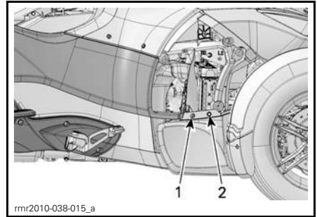
1. Vis de fixation supérieure 2. Rivet de plastique supérieur
