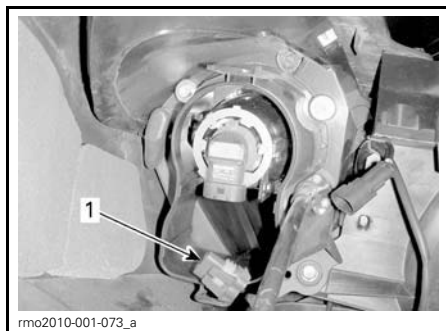
1. Connecteur débranché
