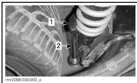
1. Régleur de came 2. Cliquet et rallonge
