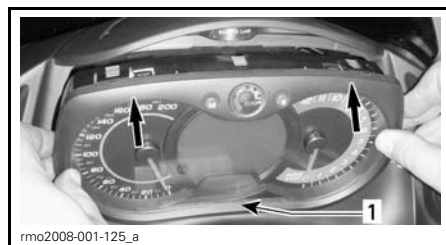
INSTALLATION DU TABLEAU DE BORD 1. Insérez le rebord inférieur d'abord puis appuyez sur le rebord supérieur
