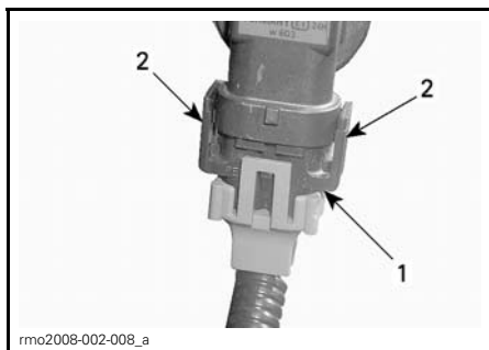
1. Connecteur d'ampoule 2. Pattes
