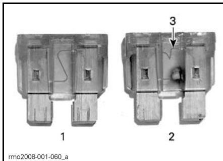
FUSIBLE SITUADO BAJO LA CUBIERTA DE SERVICIO
