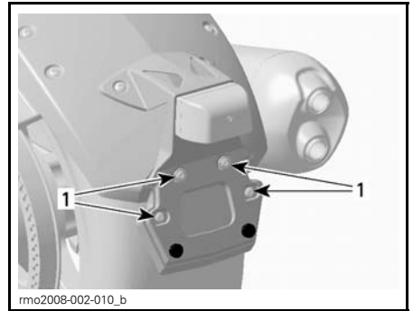
SUPLEMENTO DE AMORTIGUACIÓN (N/P 293 740 028)
