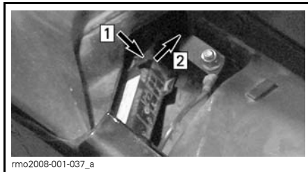
APERTURA DE LA CAJA DE FUSIBLES SITUADA BAJO EL ASIENTO
