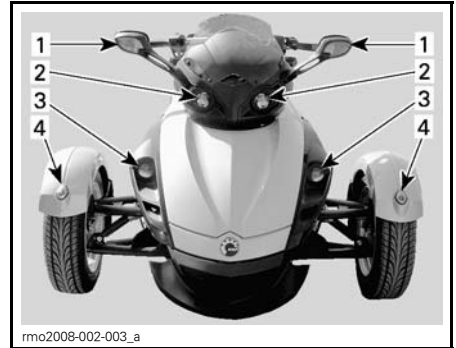
UBICACIÓN DE LAS LUCES — PARTE DELANTERA DEL VEHÍCULO
