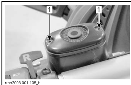
1. Tornillo en la parte superior del depósito
