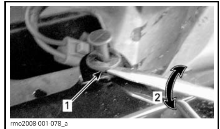
1. Tournevis plat sous la tête du rivet 2. Tournez le tournevis de 1/4 de tour
