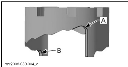
A. Mjuk fjädring (läge 1) B. Hård fjädring (läge 5)
