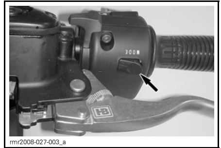
FUNKTIONSLÄGESKNAPP (M)
