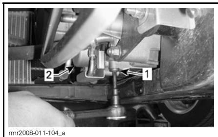
1. Motorns oljdräneringsplugg 2. Oljefilterlock
