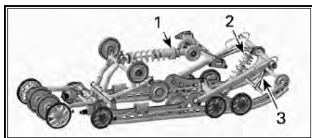
ТИПОВОЙ ВАРИАНТ — ЗАДНЯЯ ПОДВЕСКА PPS-5900A И PPS-6900A
