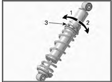
РЕГУЛЯТОР КУЛАЧКОВОГО ТИПА — АМОРТИЗАТОР НРГ
