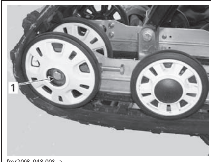
1. Болт крепления правого заднего натяжного катка
