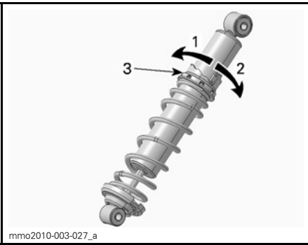
AMORTISSEUR HPG- À CLIQUET DE RÉGLAGE 1. Diminution de la tension 2. Augmentation de la tension 3. Cliquet de réglage de tension du ressort
