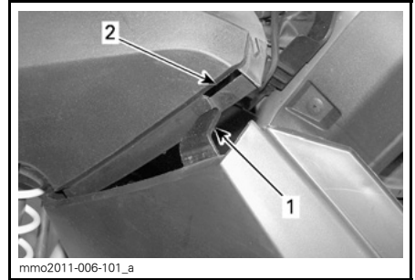
1. Languette du flanc inférieur 2. Encoche du pan inférieur
