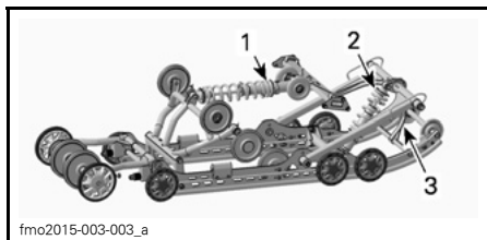
TIPIQUE - SUSPENSION ARRIÈRE PPS-5900A ET PPS-6900A
