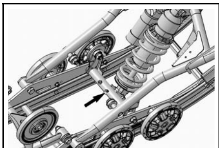
RACCORDS DE GRAISSAGE PPS2 TYPIQUES (AVANT)
