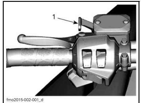
fmo2015-002-001_d TYPIQUE 1. Manette de frein de stationnement.
