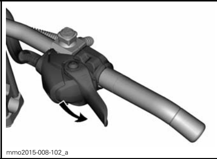
mmo2015-008-102_a ATTIVAZIONE CON IL POLLICE: PREMERE IN AVANTI PER FAR RUOTARE IL SUPPORTO DELL'ACCELERATORE
