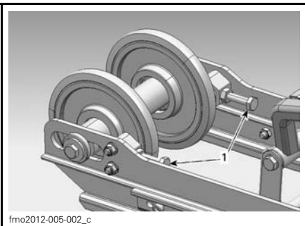
1. Justerings-skrueene
