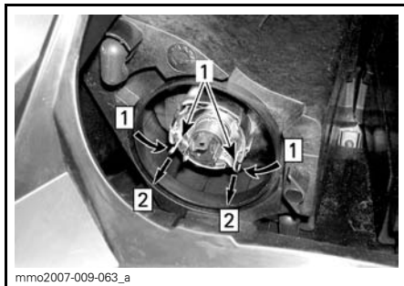
Steg 1: Trykk begge sider inn Steg 2: Dra for å løsne
