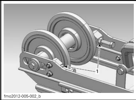
1. Justeringsboltens låsemutter
