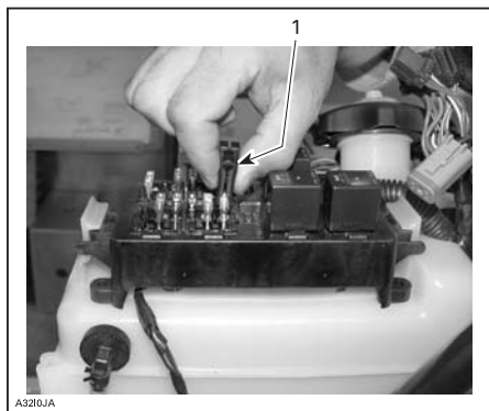
1. Säkringsborttagare/installerare
