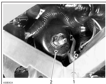
1. Polttimon liitin 2. Kumisuoja
