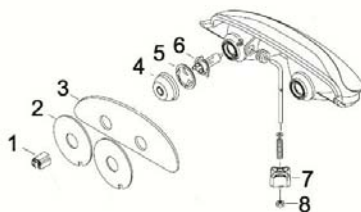
1. Polttimon liitin 2. Muovilevy 3. Suodatin 4. Kansi 5. Polttimon pidin 6. Polttimo 7. Säätonuppi 8. Elastinen lukkomutteri M6
