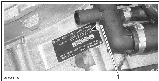
1. Moottorin sarjanumero
