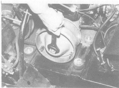
Säätökopan poistaminen Borttagning av viktkåpa
