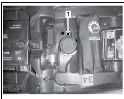
1. Réservoir de liquide de frein arrière
