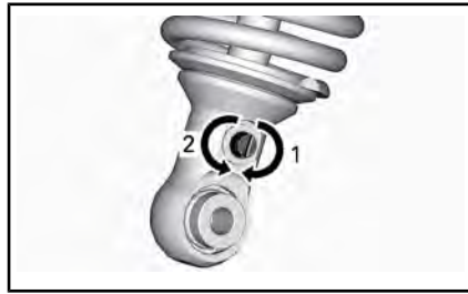
RETURSTØTDEMPING – BUNN AV STØTDEMPERE
