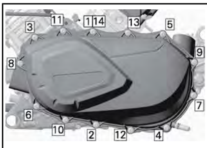
REKKEFØLGE FOR STRAMMING AV CVT-DEKSEL
