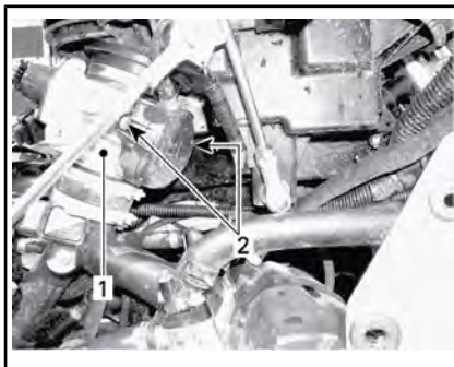
1. Carter de papillon 2. Vis du couvercle latéral
