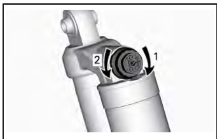
AMORTISSEMENT DE COMPRESSION - DESSUS DE L'AMORTISSEUR
