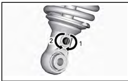
AMORTISSEMENT DES REBONDS - DESSOUS DE L'AMORTISSEUR
