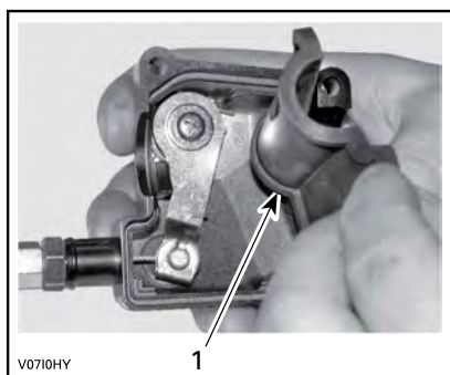
1. Protecteur de logement interne
