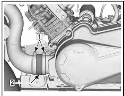
ОТСОЕДИНИТЕ ВПУСКНОЙ ВОЗДУХО-ВОД ВАРИАТОРА
