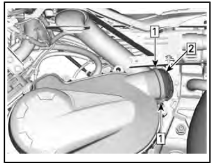
SCOLLEGAMENTO DEL CONDOTTO DI USCITA ARIA CVT
