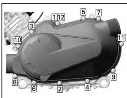
SEQUENZA DI SERRAGGIO DELLA CARENATURA DELLA CVT
