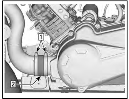
SCOLLEGAMENTO DEL CONDOTTO DI INGRESSO ARIA CVT
