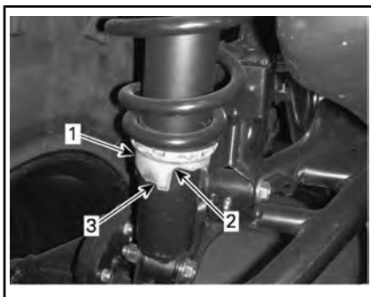
ПРИСПОСОБЛЕНИЕ ДЛЯ РЕГУЛИРОВКИ
