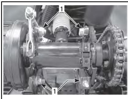
TYPISCH — HINTERACHSE
