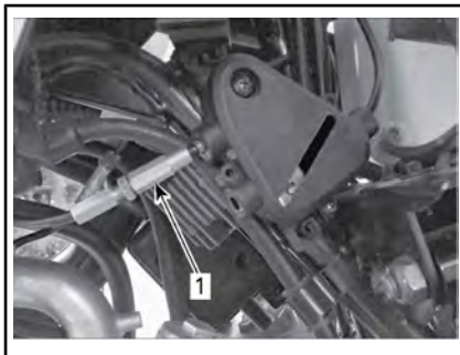
EINSTELLUNG VOM GASZUGBEGRENZUNGSFACH ZUM MOTOR
