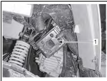
1. Ventil Lufteinspritzung
