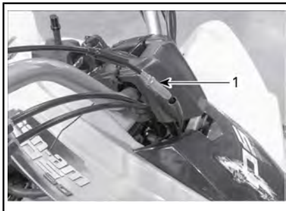
EINSTELLUNG VOM GASHEBEL ZUM GASZUGBEGRENZUNGSFACH
