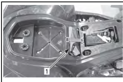
1. Werkzeugsatz
