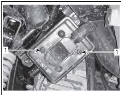
1. Schrauben entfernen
