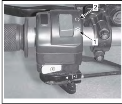
TYPISCH - MOTOR-NOTHALT-SCHALTER
