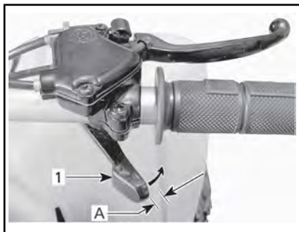
TYPISCH — NORMALES SPIEL
