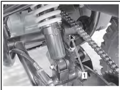
1. Führungsrollen Antriebskette
