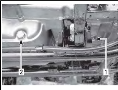
ABLASSSCHRAUBE — LINKE MOTORSEITE
