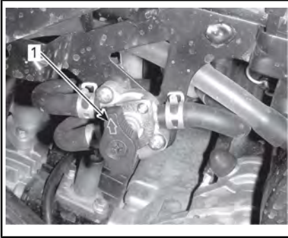
LINKE SEITE DES FAHRZEUGS
