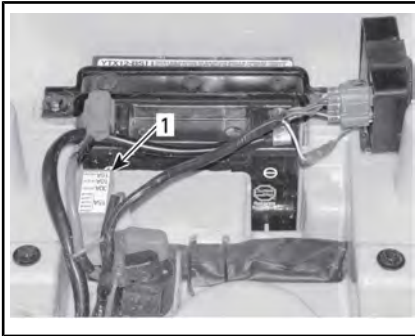
1. Держатель предохранителей.
