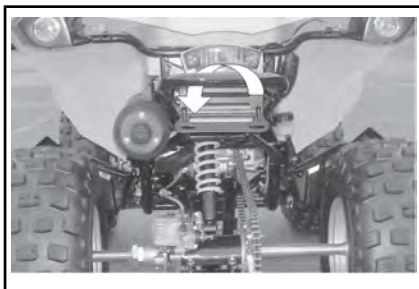
МЕСТО КРЕПЛЕНИЯ РЕМНЯ НА ЗАД- НЕМ БАМПЕРЕ
