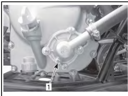
1. Пробка сливного отверстия системы охлаждения
