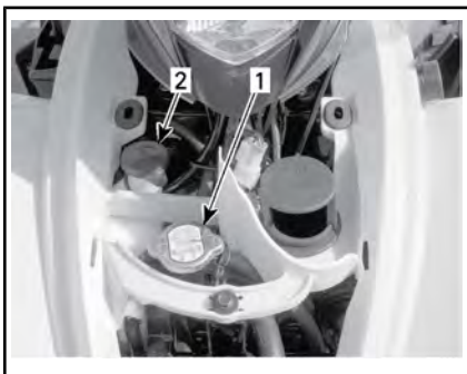
1. Крышка радиатора
