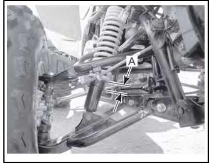
ПЕРЕДНЯЯ ПОДВЕСКА
