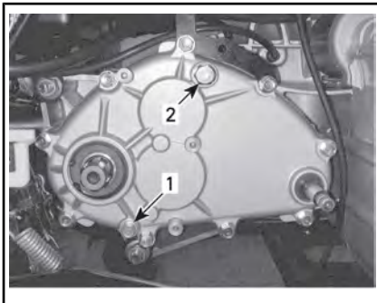
1. Пробка сливного отверстия коробки передач
