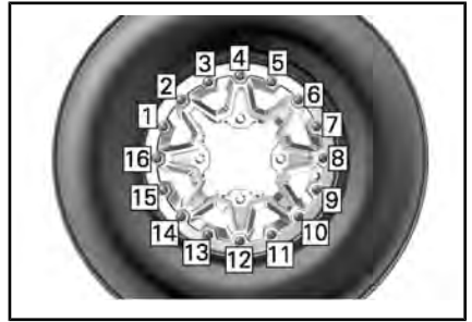
TYPIQUE - SÉQUENCE DE SERRAGE FINAL
