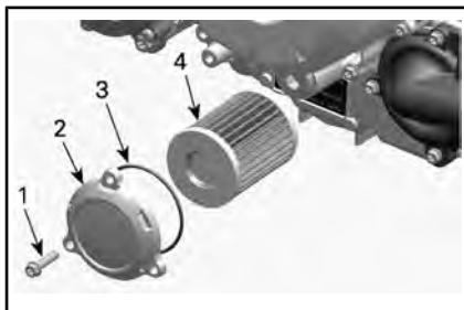
TYPIQUE - PIÈCES RETIRÉES POUR PLUS DE CLARTÉ
