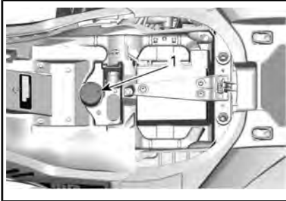
1. Réservoir de liquide de frein arrière
