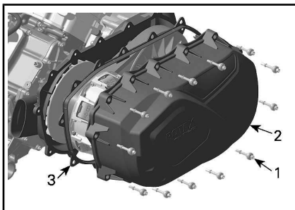
1. CVT-dekselschroef
