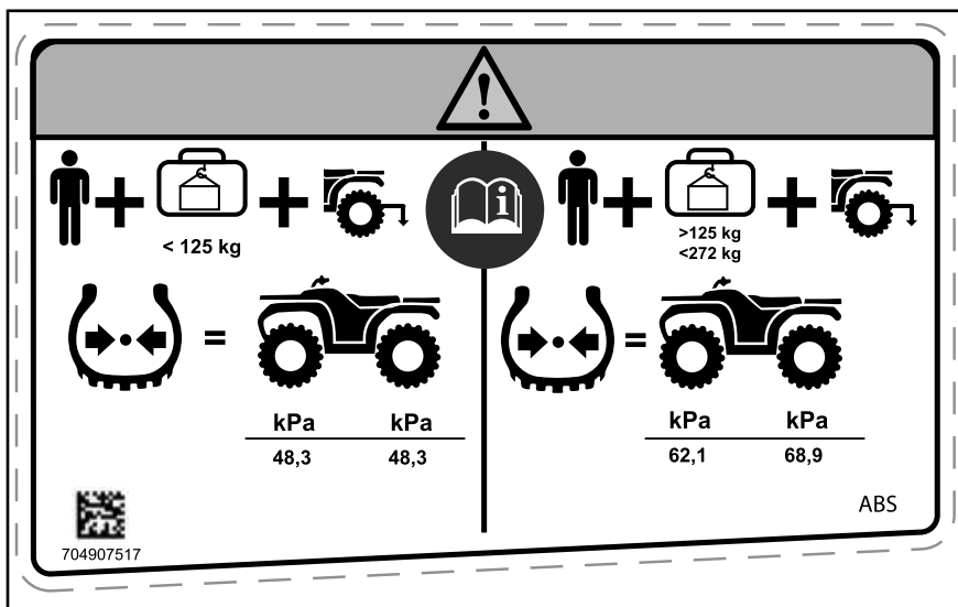
LABEL 5 - 2-UP MODELLEN MET ABS
