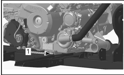
1. Afvoerplug
