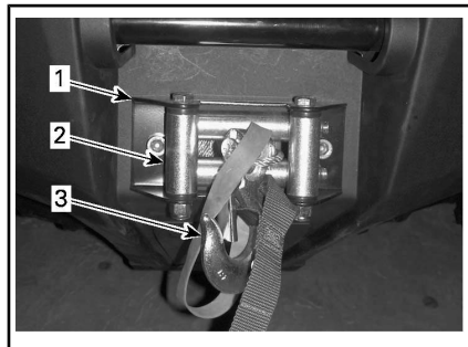
1. Lier 2. Kabelgeleider met rollen 3. Lierhaak
