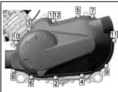
SEQUENZA DI SERRAGGIO DELLA CARENATURA DELLA CVT
