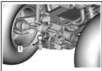
1. Gancio di traino
