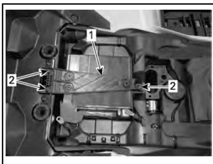
1. Support de batterie 2. Vis de fixation
