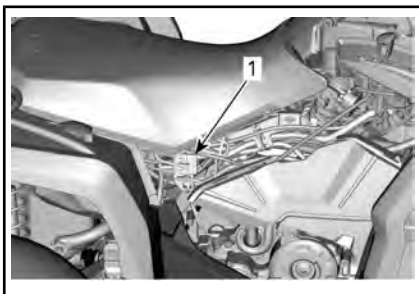
1. Porte-fusibles arrière et éléments fusibles
