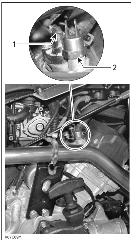
1. Vite di spurgo 2. Sensore di temperatura del motore
