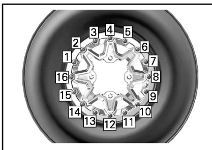
TÍPICO - SEQUÊNCIA FINAL DE APERTO
