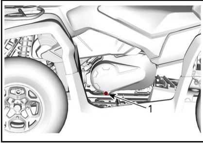
1. Tapón de drenaje de la CVT
