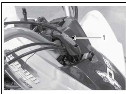
AJUSTE DA ALAVANCA DO ACELERADOR À CAIXA LIMITADORA DO ACELERADOR
