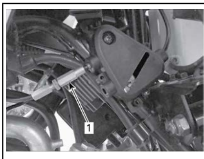
AJUSTE DA CAIXA LIMITADORA DO ACELERADOR AO MOTOR
