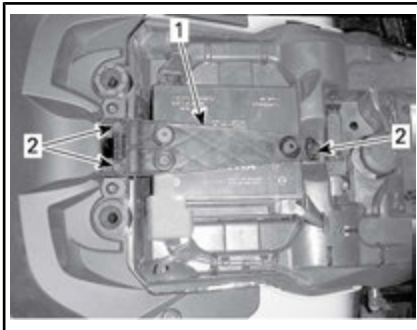
1. Fascetta di fissaggio della batteria 2. Viti di bloccaggio
