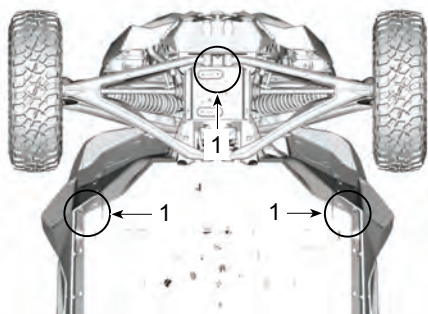
前部千斤顶支架位置
