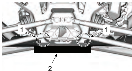
后部液压千斤顶为止
