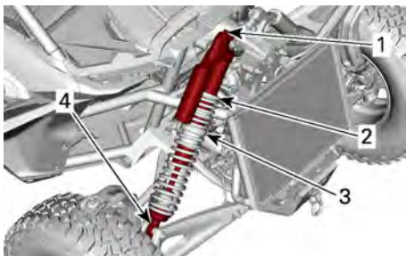
典型示例 - 前悬架
